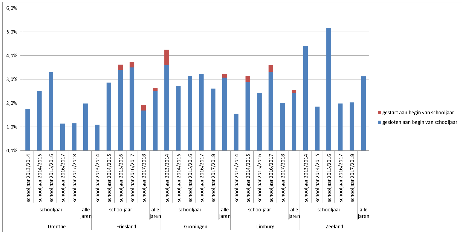
Figuur 3. Aantal sluitingen per schooljaar en het gemiddelde aantal sluitingen van de afgelopen 5 schooljaar, voor de provincies Drenthe, Friesland, Groningen, Limburg en Zeeland.
